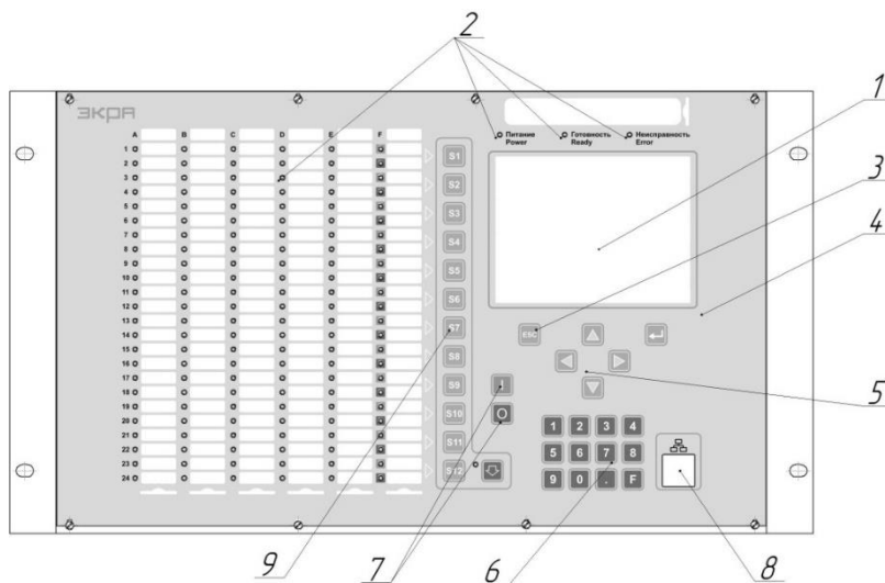
б) терминал типа ЭКРА 2X3(A)
