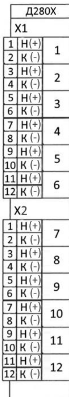
Рисунок Б.1.2 – Схема подключения блока типа Д280Х
