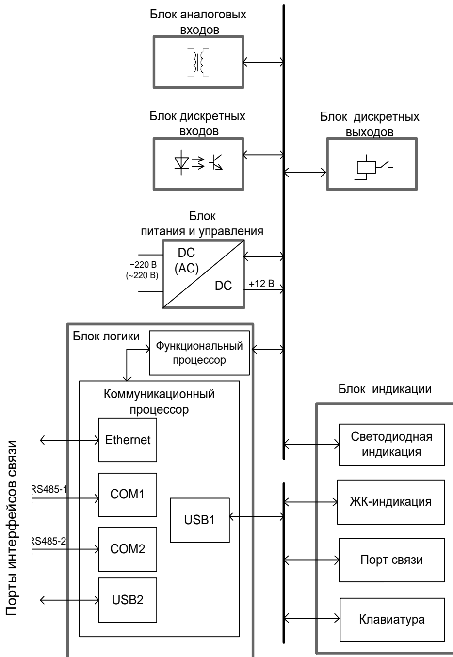
Рисунок Г.1 – Базовая 1) блок-схема терминалов типов ЭКРА 2Х1(А), ЭКРА 2Х2(А), ЭКРА 2Х3(А), ЭКРА2Х7(А)
