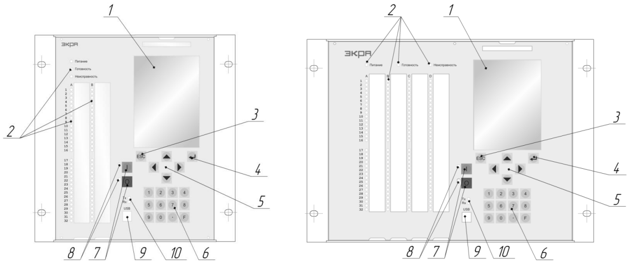
б) терминал типа ЭКРА 2X2(A)
