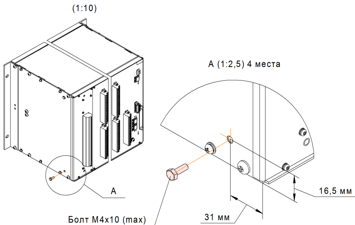
Рисунок А.5 – Дополнительные места крепления терминалов типов ЭКРА 2X1(A) – ЭКРА 2X3(A), ЭКРА 2X5(A), 2X6(A) 1)
