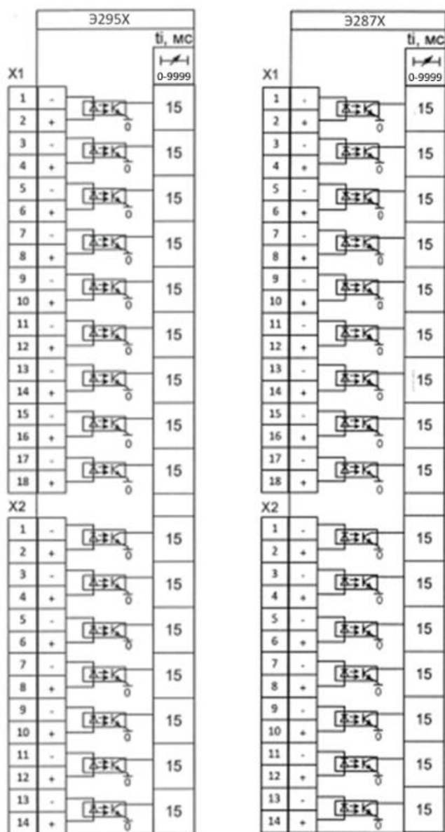
Рисунок Б.2.2 – Схемы подключения блоков типа Э295Х и Э287Х
