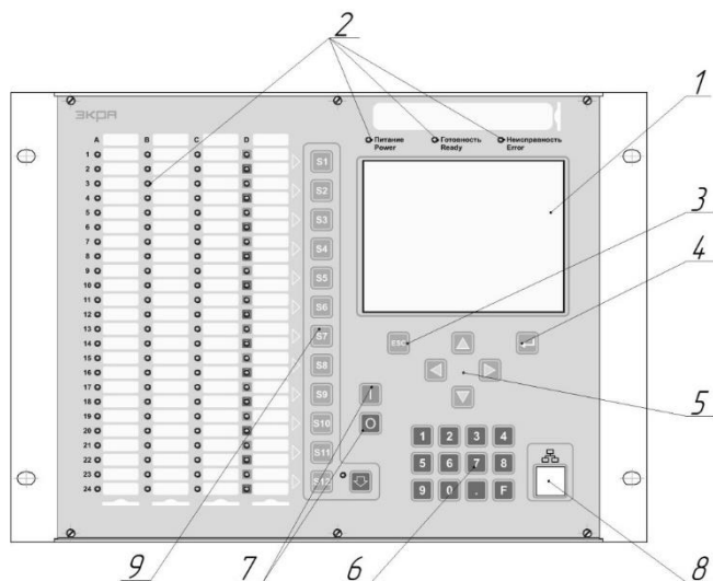
а) терминал типа ЭКРА 2X2(A)
