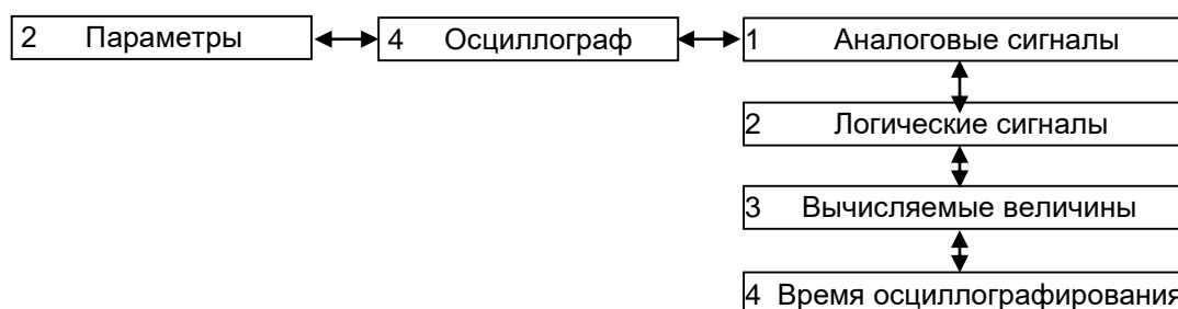
Рисунок 30 – Структура меню Осциллограф
